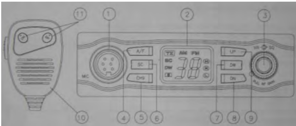
Рис. 1. Органы управления и отображения MJ-200Plus
