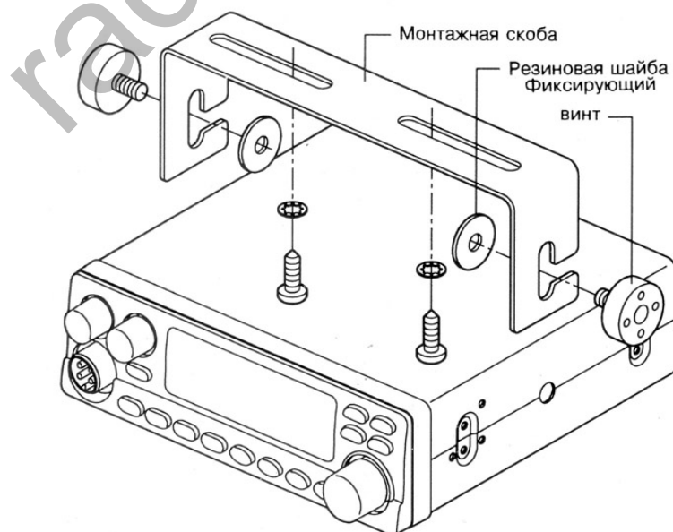
Рис.2. Крепление радиостанции при помощи монтажной скобы.
